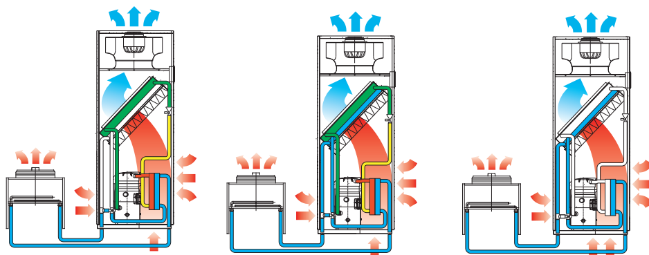
Fig. A 单一机械制冷
